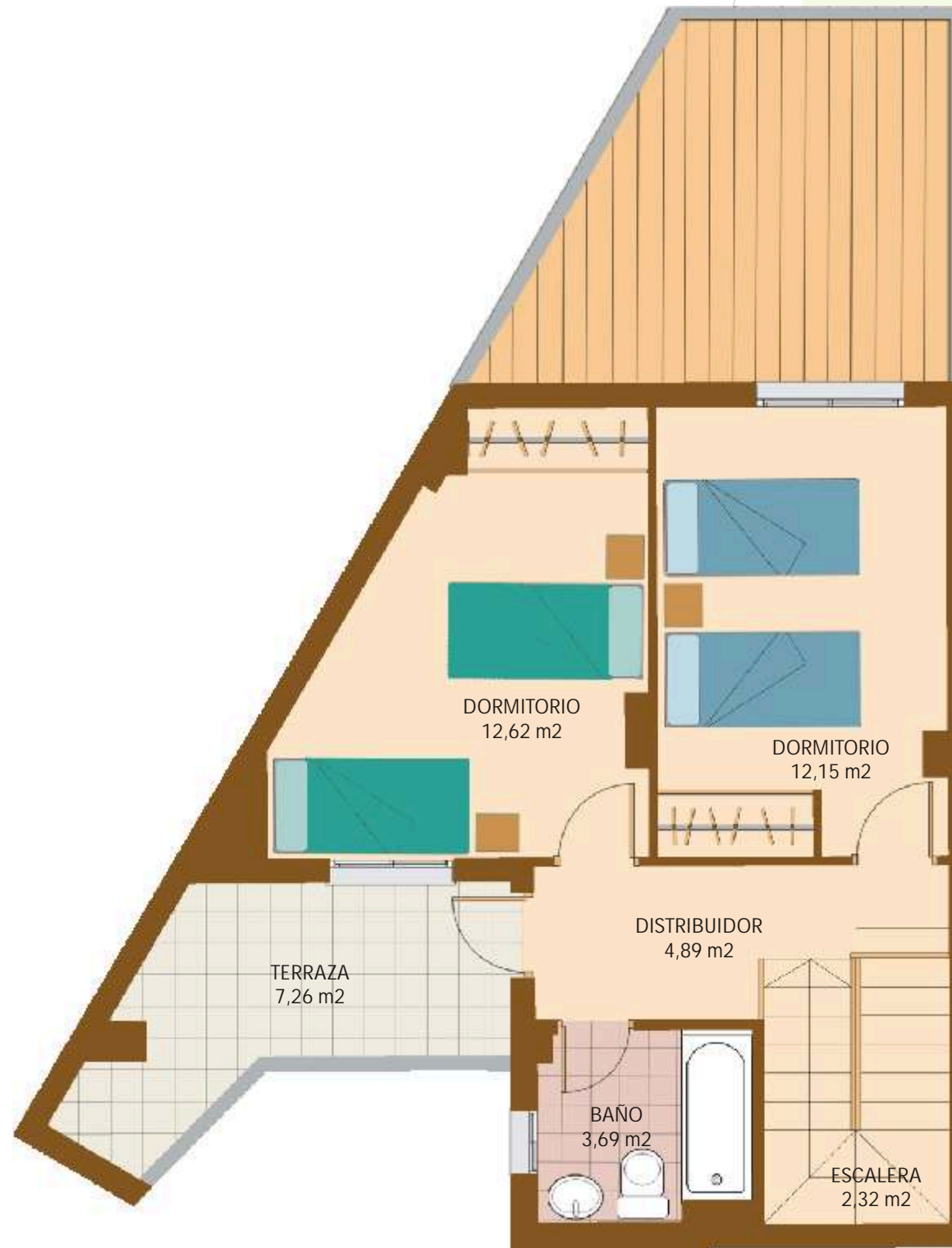
BAJO CUBIERTA
