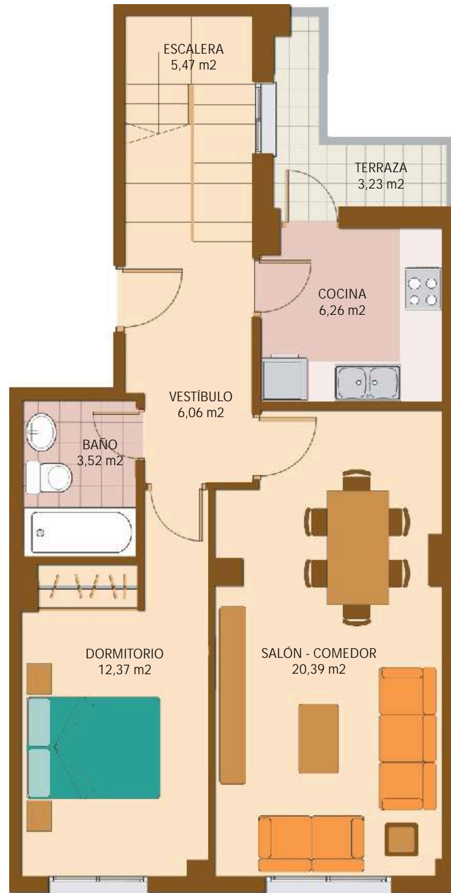
PLANTA PRIMERA
