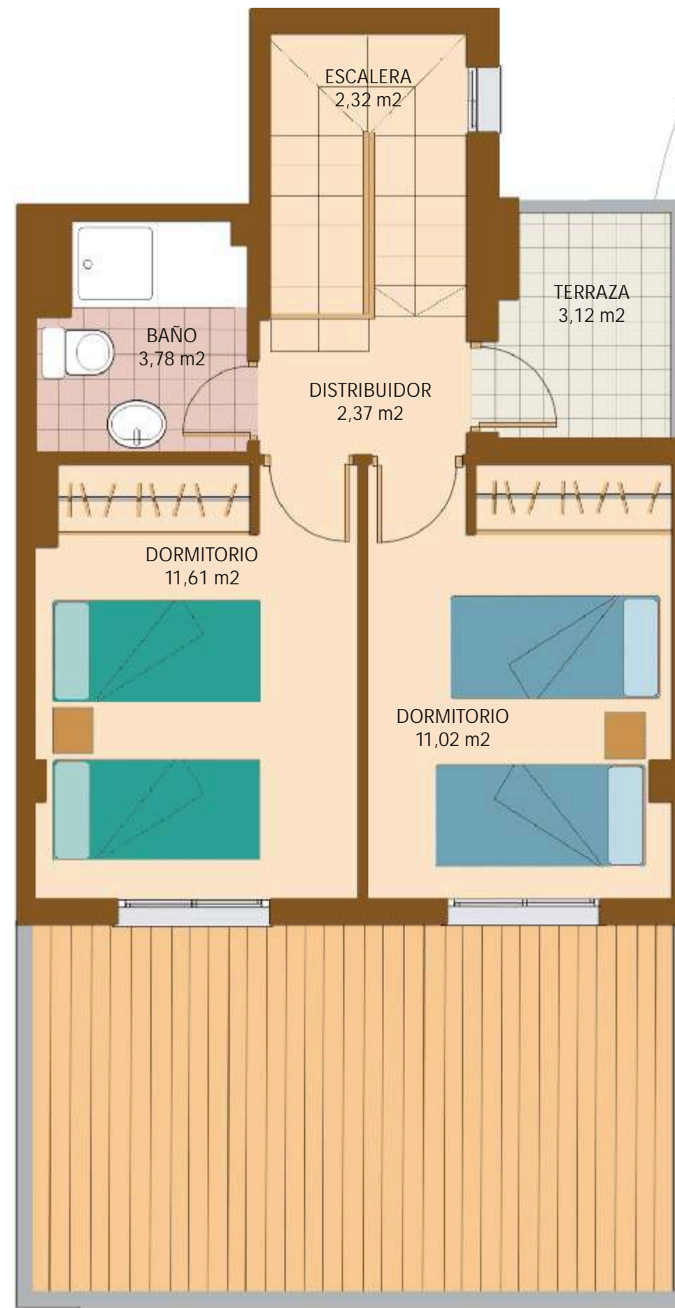
BAJO CUBIERTA
