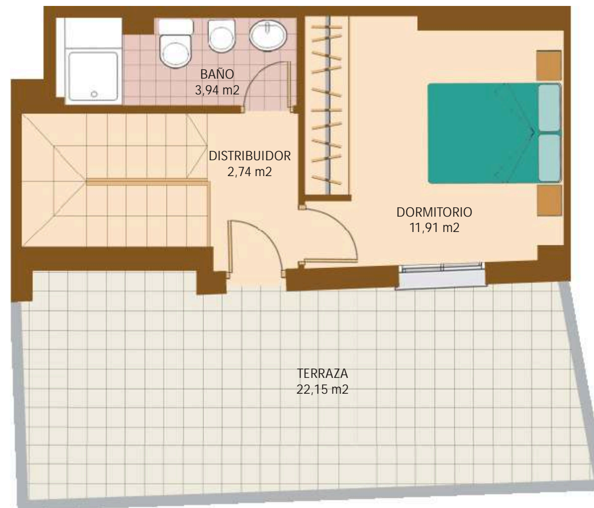
BAJO CUBIERTA
