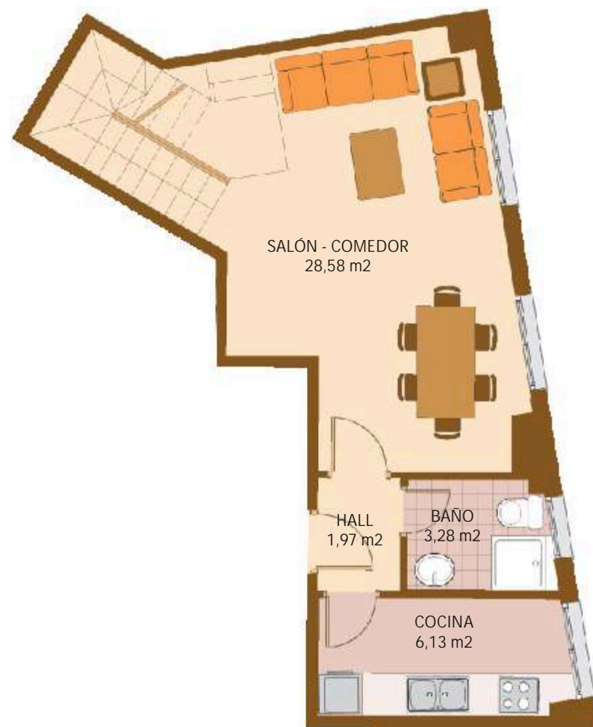
PLANTA PRIMERA
